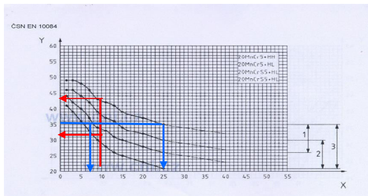
Pás prokalitelnosti oceli 20MnCr51. HH min. až HH max.;2. HL min. až HL max.;3. H min. až H max.
