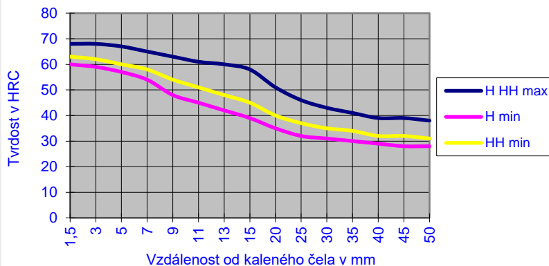
Pás prokalitelnosti
